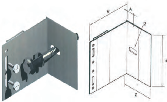
STAFFA NORMALE
