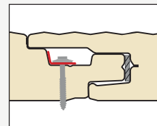
Particolare - Fissaggio nascosto UniWall
